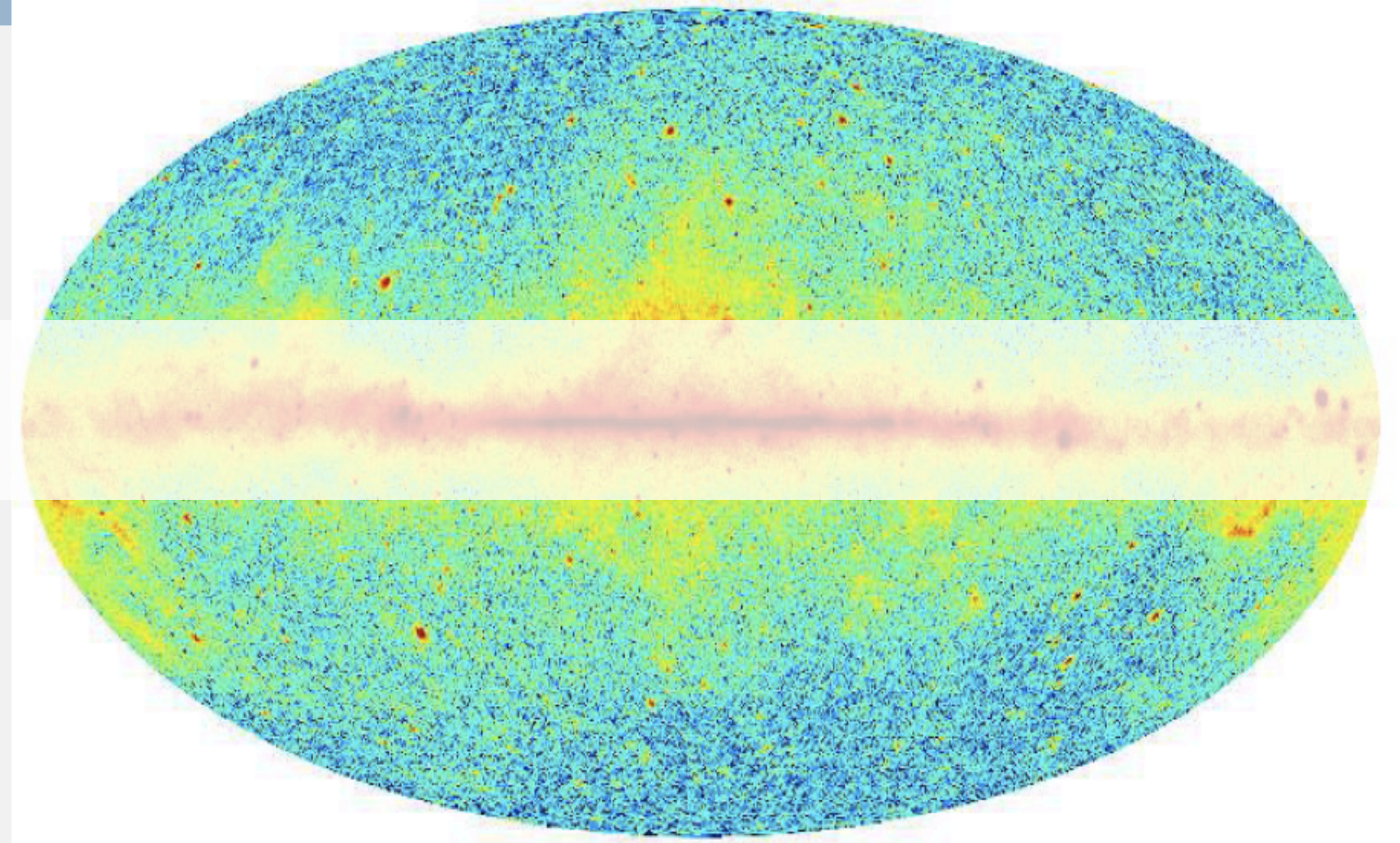
Fermi-LAT 1–2 GeV
